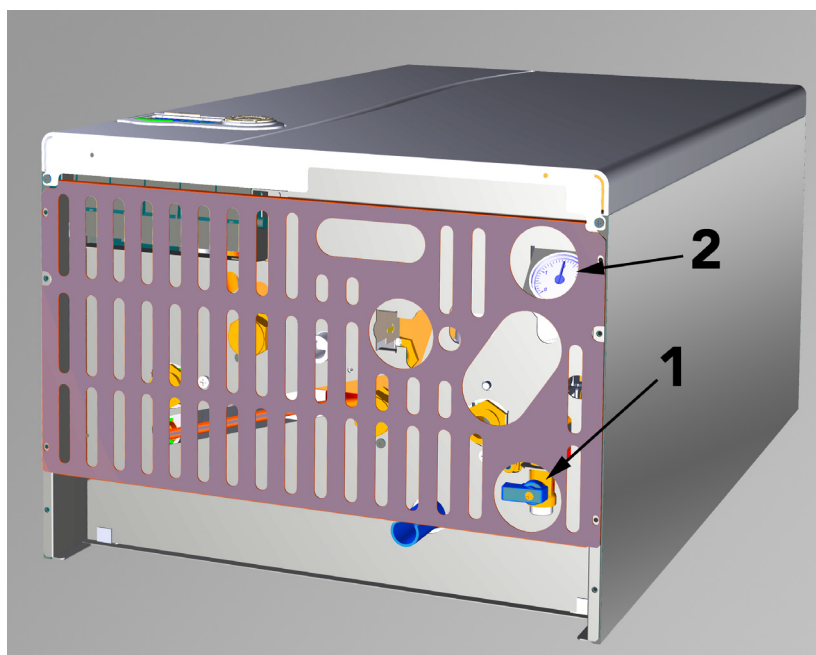
fig. 16 - Torneira de enchimento
