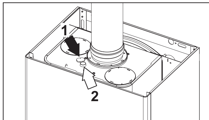
fig. 28 - Análise de fumos
