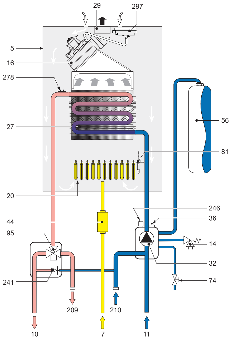
fig. 31 - Circuito hidráulico
