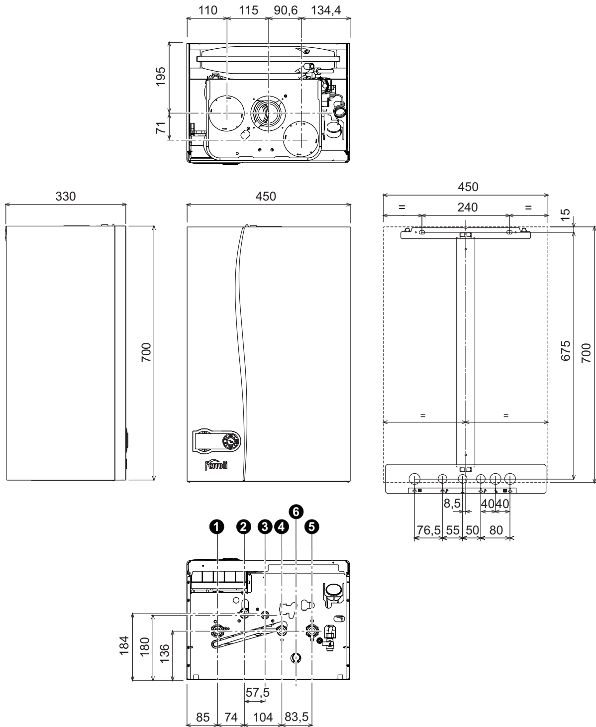
fig. 29 - Dimensiones y conexiones
