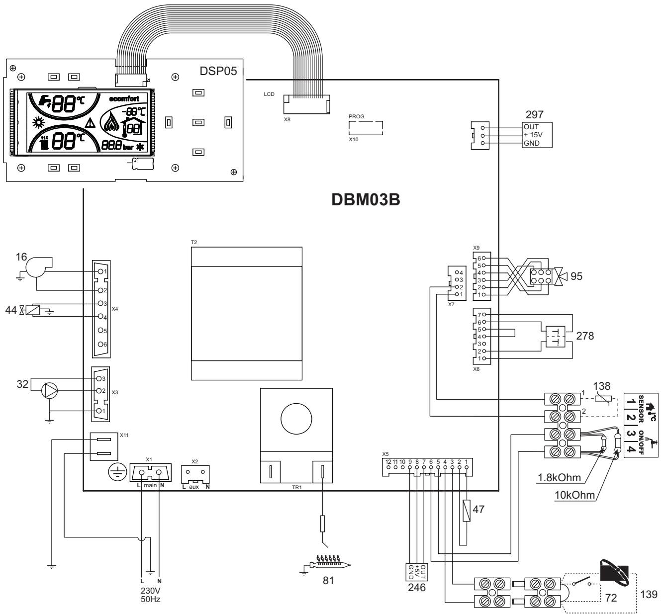
fig. 32 - Esquema eléctrico
