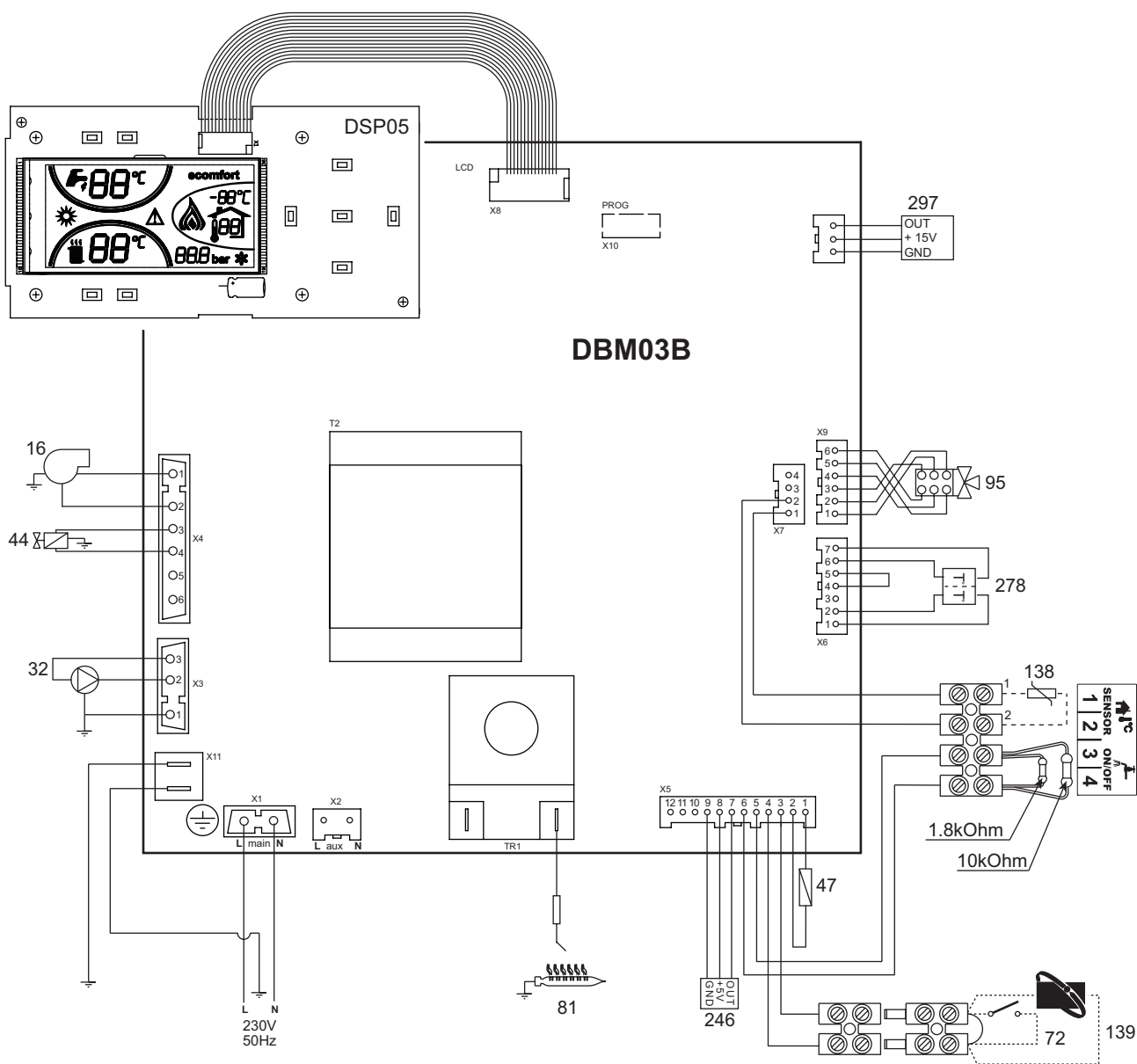
fig. 32 - Esquema eléctrico
