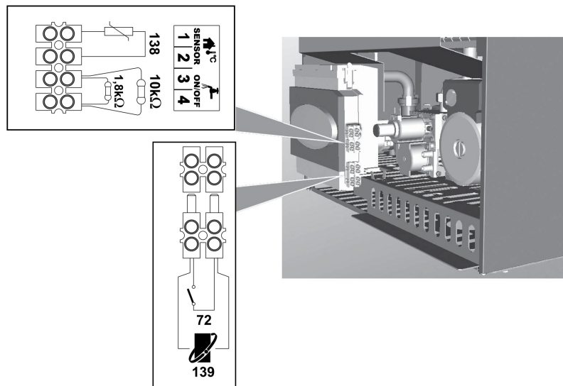
fig. 18 - Acesso à régua de terminais eléctrica
