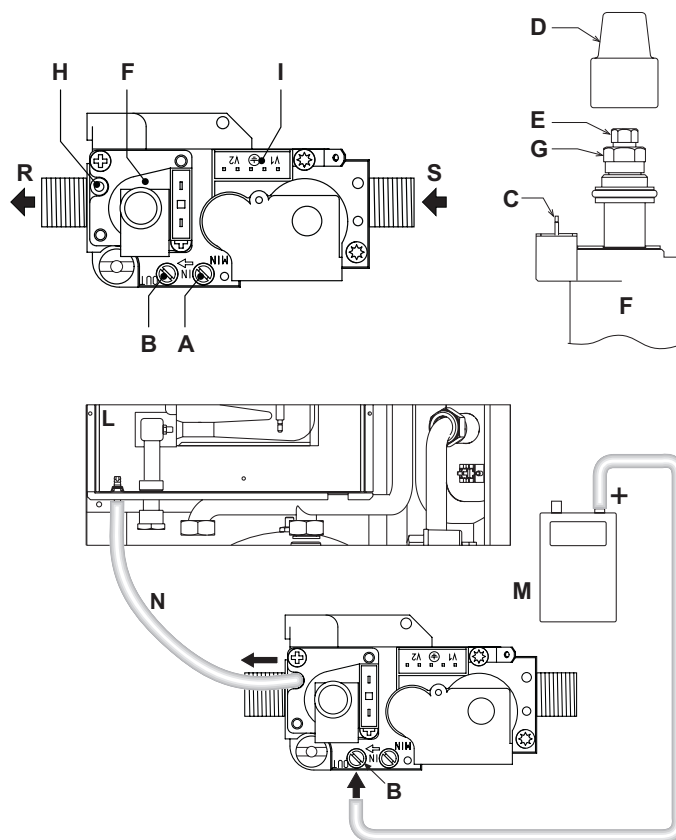
fig. 26 - Válvula de gas
