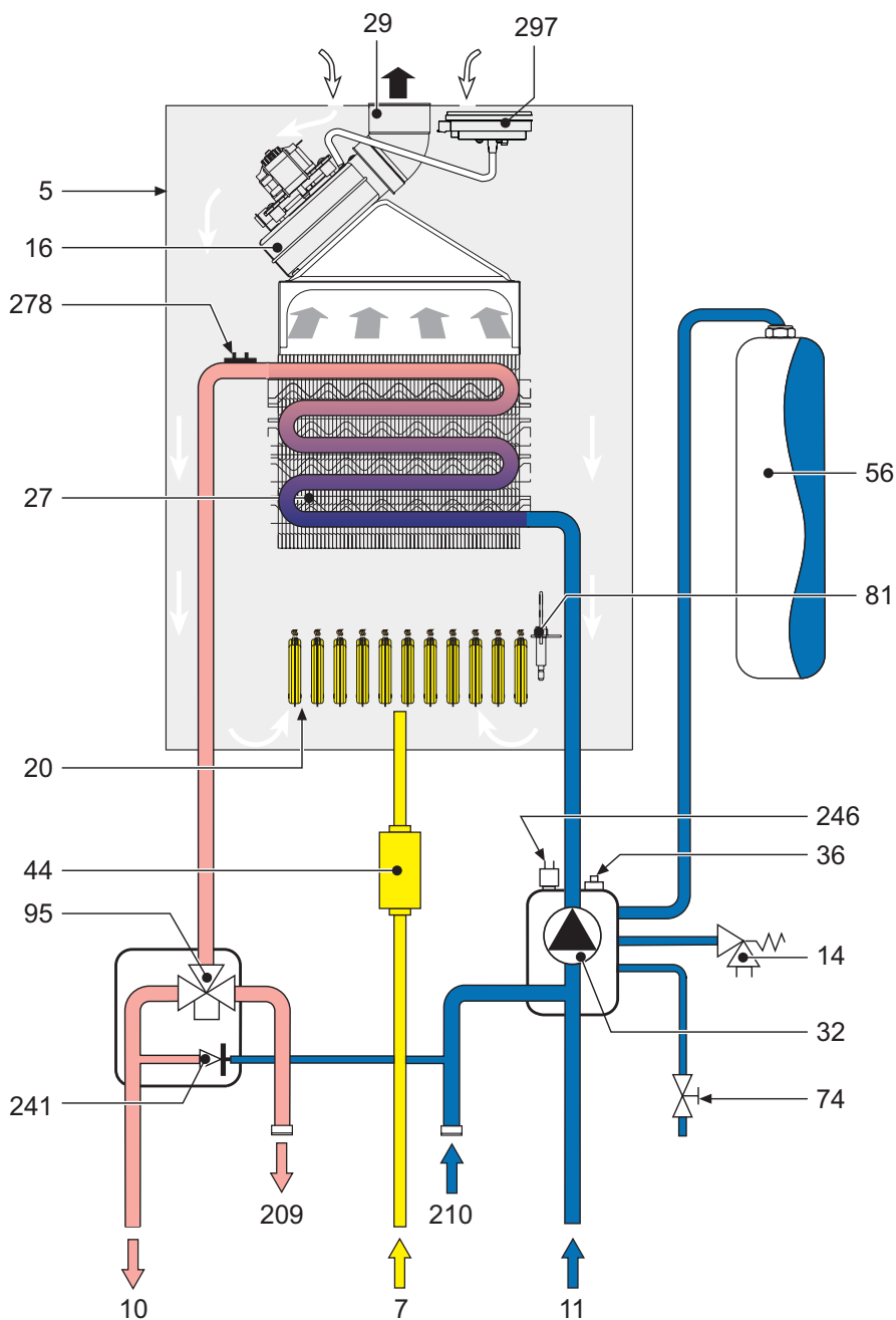
fig. 31 - Circuito hidráulico
