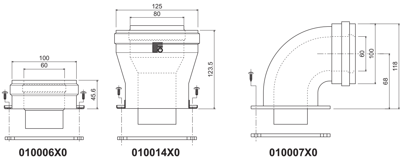
fig. 21 - Acessórios iniciais para condutas coaxiais
