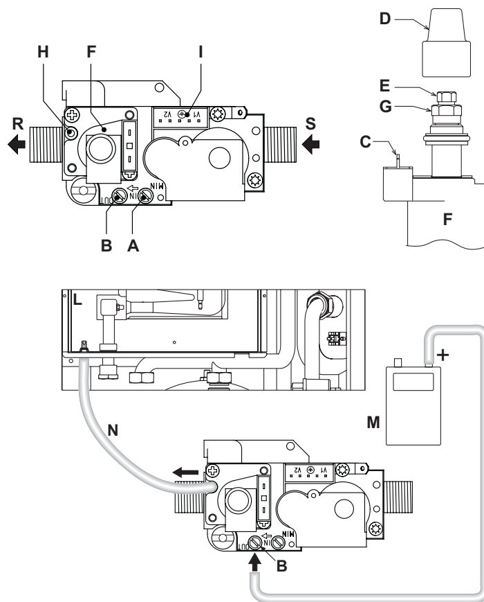
fig. 26 - Válvula de gás
