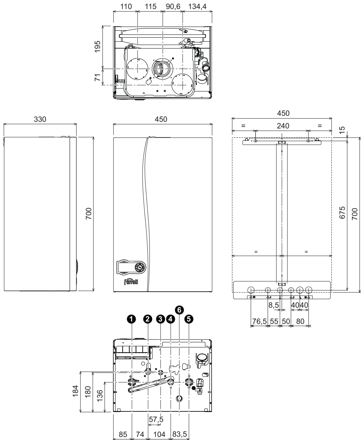
fig. 29 - Dimensioni e attacchi
