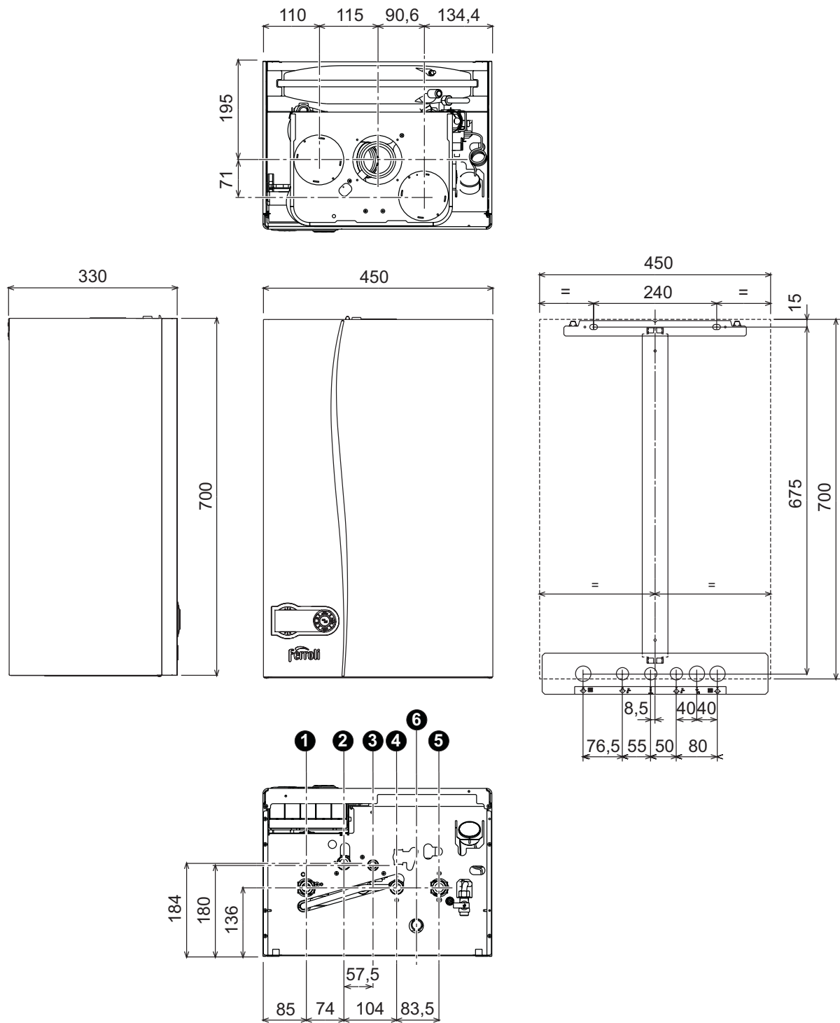
fig. 29 - Dimensões e ligações
