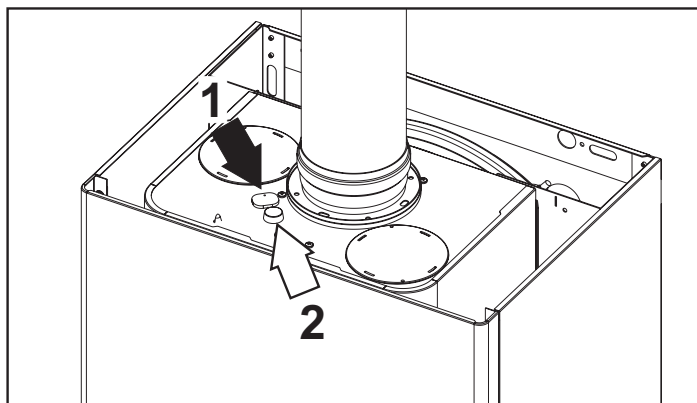
fig. 28 - Análisis de los humos
