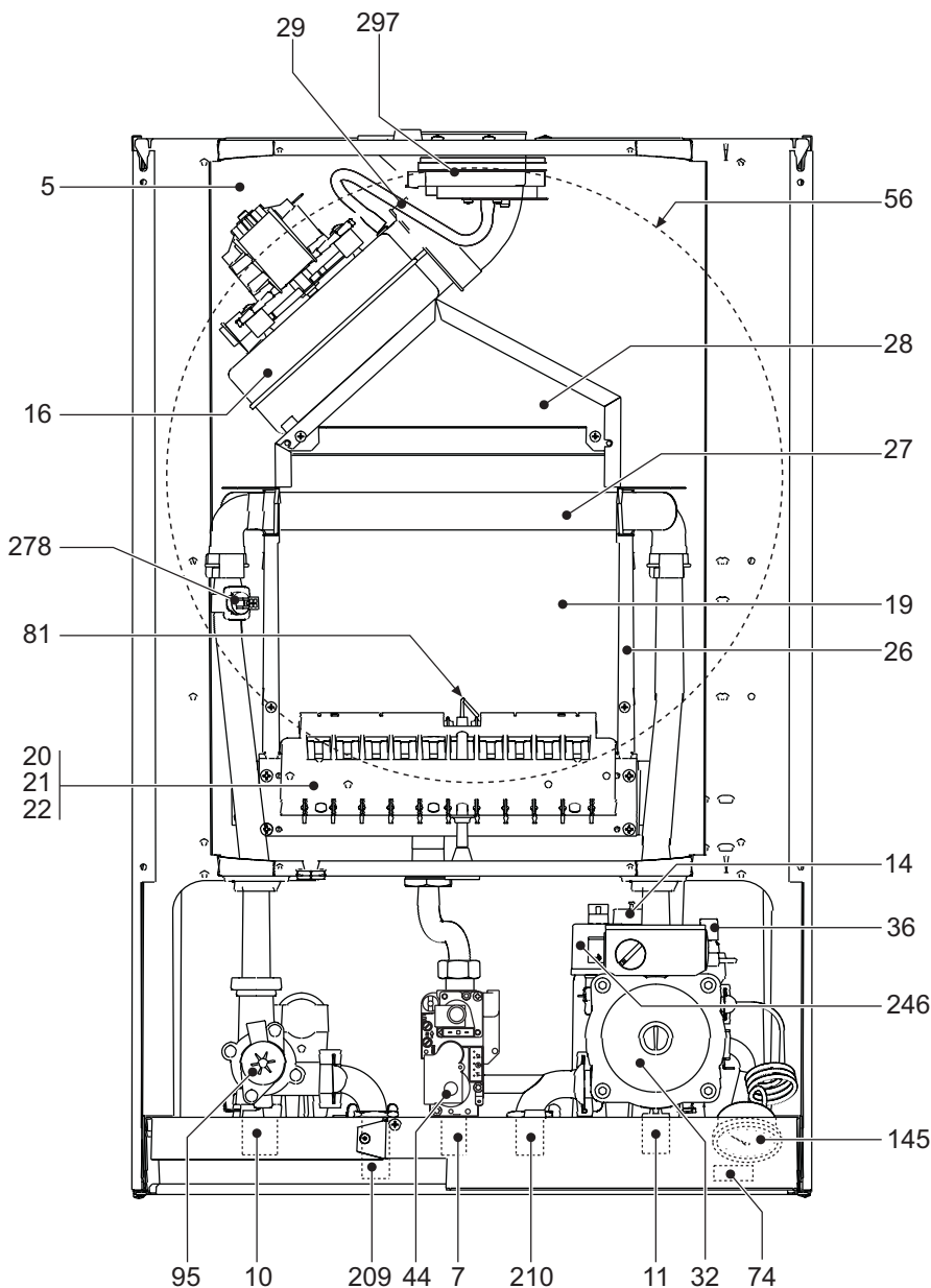
fig. 30 - Vista general
