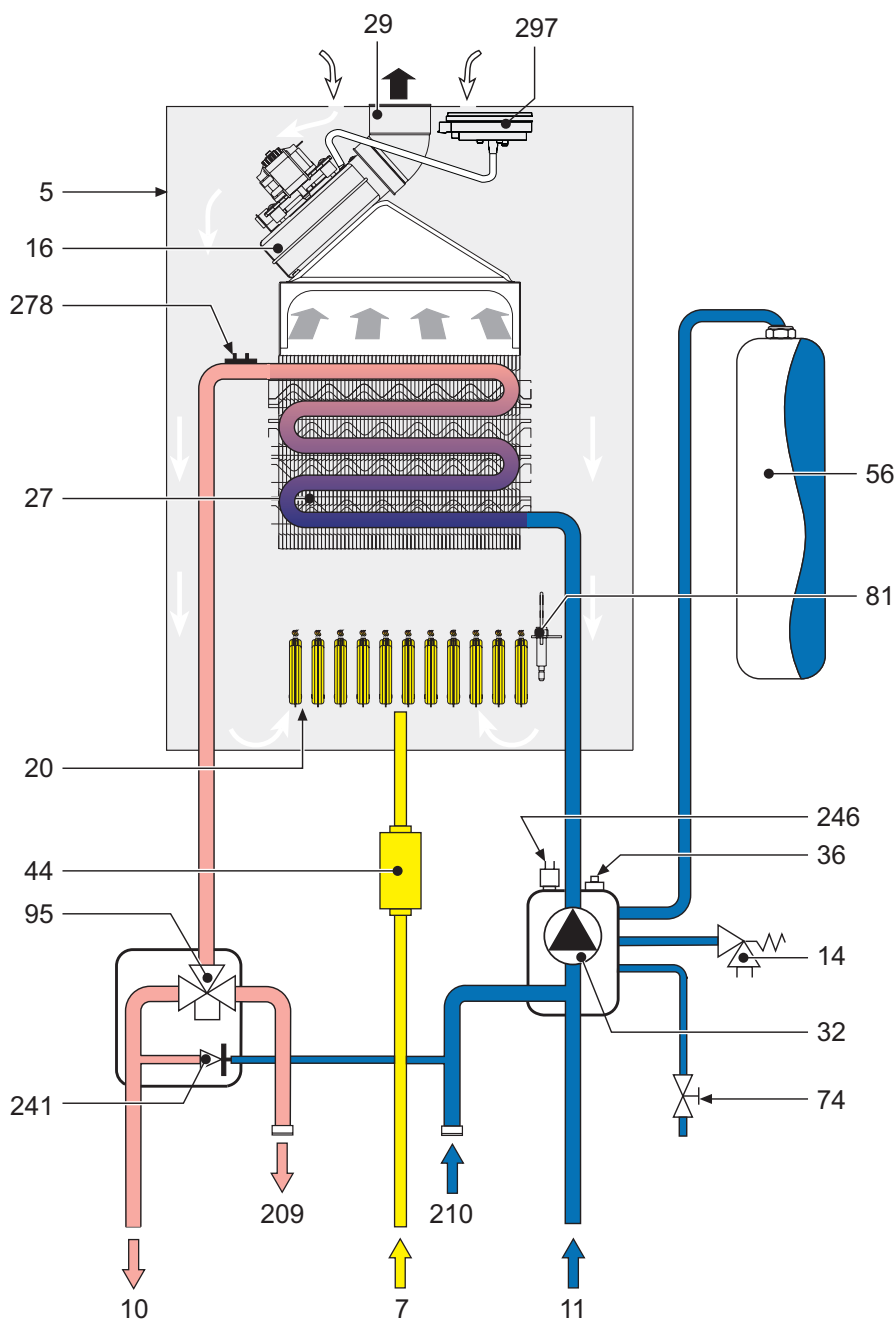
fig. 31 - Circuito idraulico
