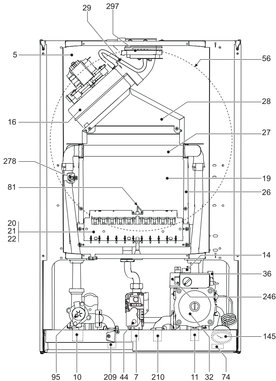
fig. 30 - Vista geral
