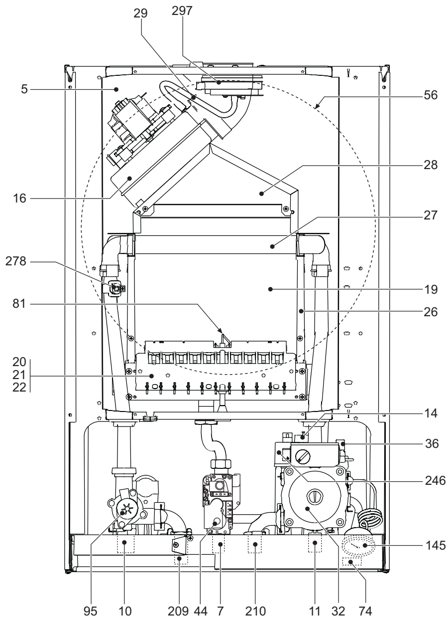
fig. 30 - Vista generale
