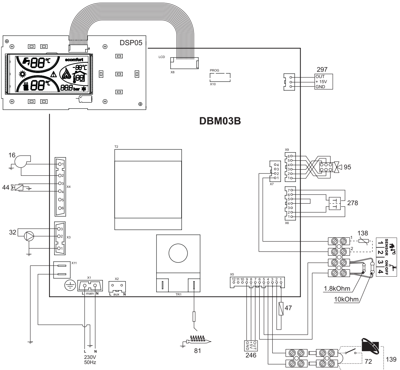
fig. 32 - Schema elettrico
